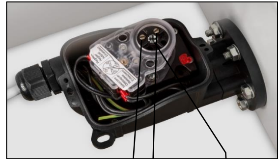
Stelschroef MC1 Stelschroef MC2 Borgschroef
