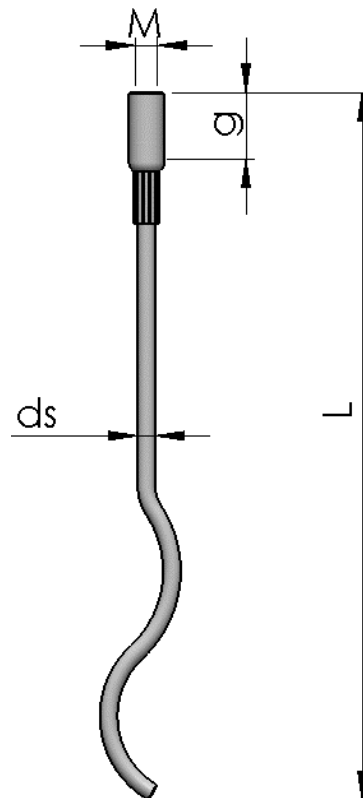
Figur 9 Transportanker med armeringsjern langbølgeskitse.
