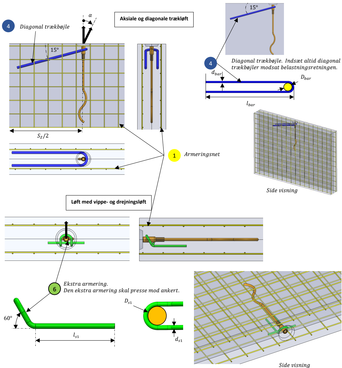
Figur 7 Armering i betonavæggen.
