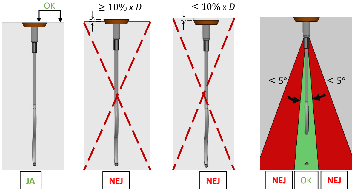
Figur 4 Korrekt placering af holdeplade.
