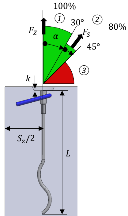
Aksiale og diagonale trækløft
