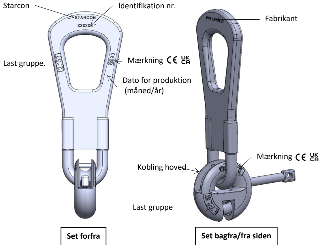
Figur 2 Mærkning på ringkobling.
